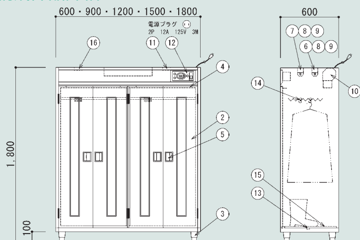
※図面はOC-150型です。OC-150型より扉が2箇所になります。
