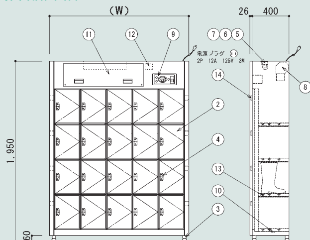
※図面はOS-45型です。
