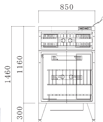
※図面はDS-113型です。
