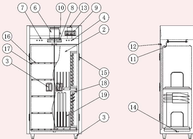
図: IHDS (K) -10型
