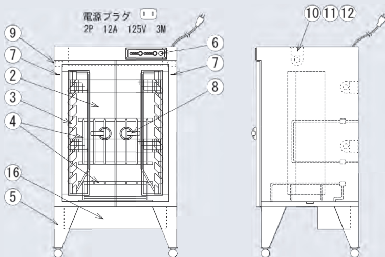
図:DS-113型
