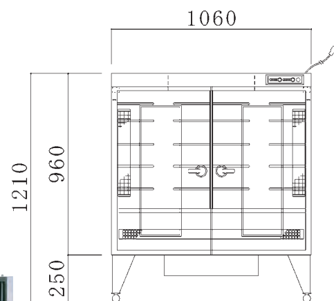
※図面はDS-115B型です。
